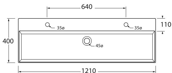
Bovenaanzicht
