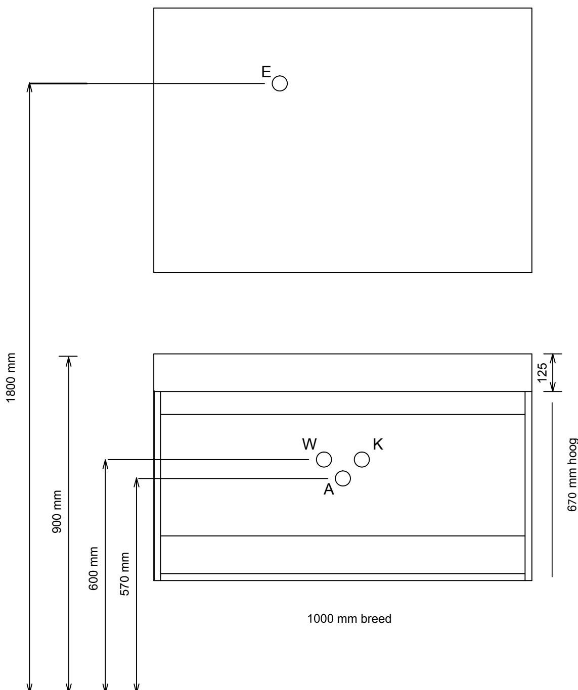
Vooraanzicht
