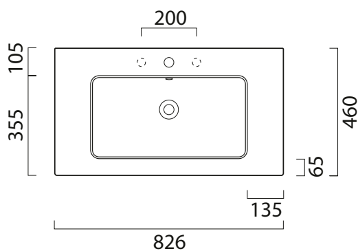
Bovenaanzicht
